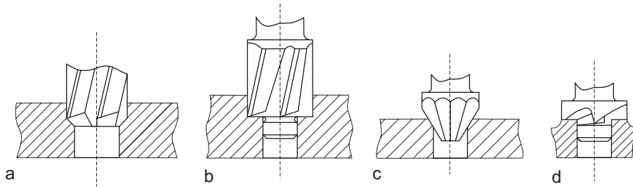
a, b, c, d - razni oblici (razne površine) upuštača prema obliku obrađivane površine (rupe);
